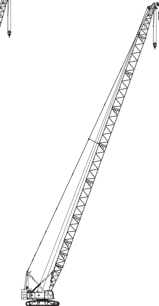
クレーン仕様 補助シーブ付きブーム最長
